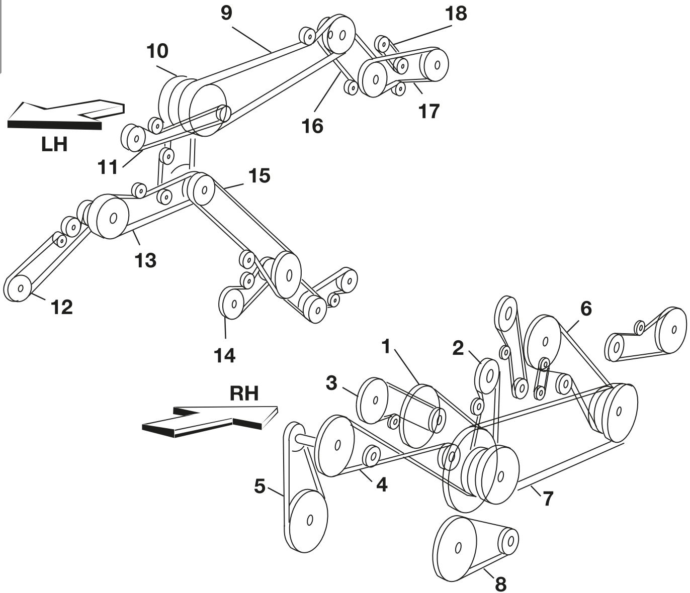
TX 62-64-65-66 (RH)
